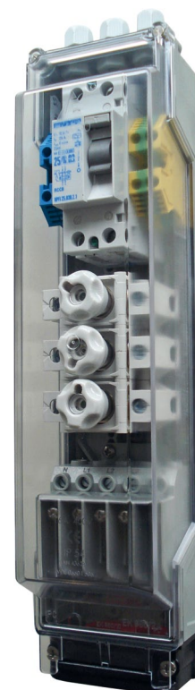
Obudowa EK 580 o długości 368 mm z przykładowym wyposażeniem
